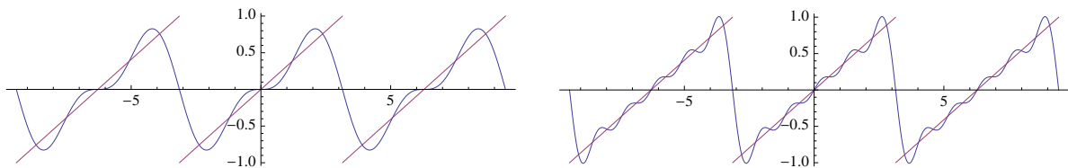
Abbildung 10.1: Zweite und fünfte Partialsumme der Fourier-Reihe.
