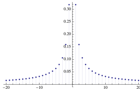
Abbildung 10.2: Beträge der Fourier-Koeffizienten.
